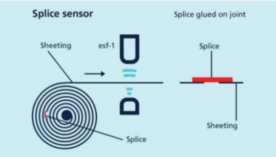
Czujnik ESF jako detektor podwójnego arkusza, zgrubień, spoin
