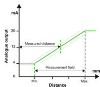
Wyjście analogowe
