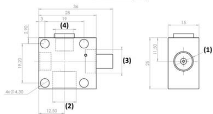
Dimensioner (mm)
