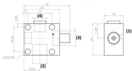
Dimensioner (mm)
