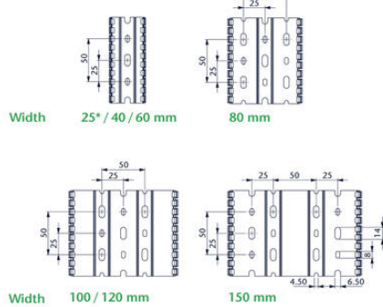
Base holes EN 50085-2-3
