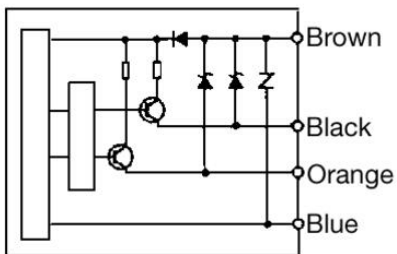
PNP output
