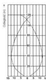
Wyczuwanie bezpośrednie NAR10-PG/NAR10F-PG
