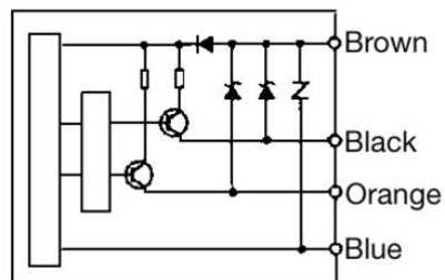
PNP output
