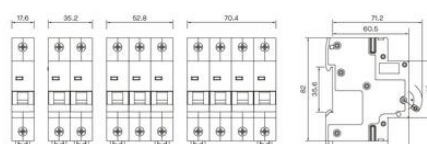
Wymiary [mm]
