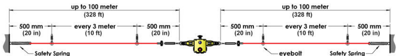
Wyłącznik linkowy GLHD ze sprężynami.
