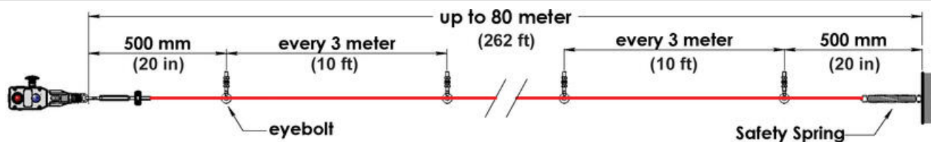
Wyłącznik linkowy GLS-SS ze sprężyną.
