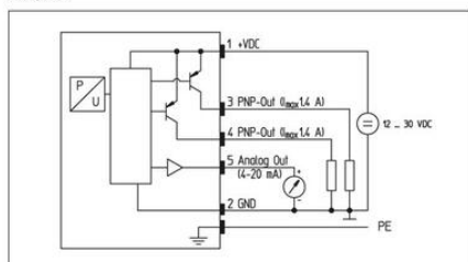
Wiring chart
