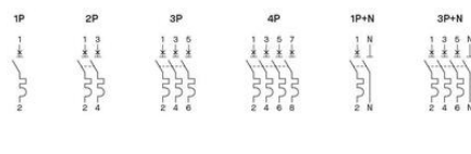
Schemat podłączenia
