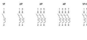
Schemat podłączenia
