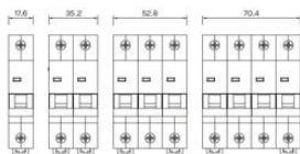
Wymiary [mm]
