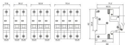
Wymiary [mm]
