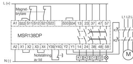
9. Tvåkanalig inkoppling av magnetbrytare. Automatisk återställning. Övervakning av externa kontaktorer (K1 och K2).
