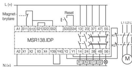
10. Enkanalig inkoppling av magnetbrytare. Övervakad manuell återställning. Övervakning av externa kontaktorer (K1 och K2).
