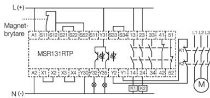
7. Enkanalig inkoppling av magnetbrytare. Automatisk återställning. Övervakning av externa kontaktorer
