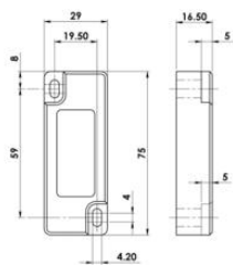
ACTUATOR
