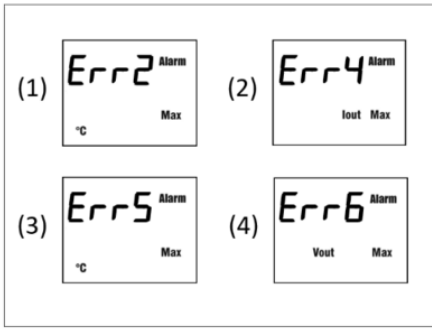
Fig. 9-3 Error codes
