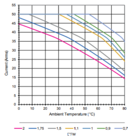
GNA - 50 A
