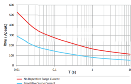
GNA - 50 A
