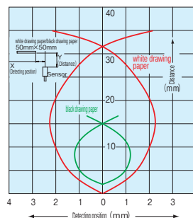
GN-Z3CR GN-Z3CRPN
