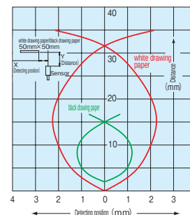
GN-Z3CR-J GN-Z3CRPN-J
