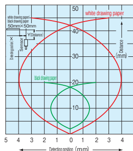
GN-Z3C GN-Z3CPN
