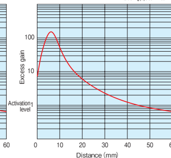
GN-Z3CR-J GN-Z3CRPN-J
