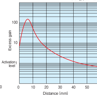
GN-Z3CR GN-Z3CRPN
