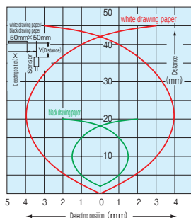
GN-Z3C-J GN-Z3CPN-J
