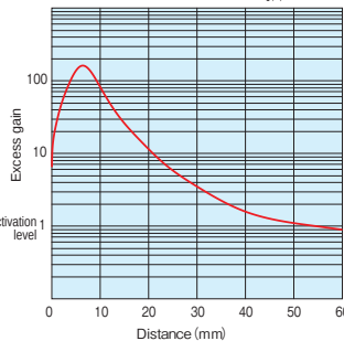
GN-Z3C-J GN-Z3CPN-J
