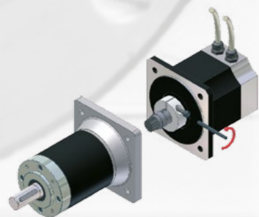
Versione con morsetto a vite Clamp disk version
